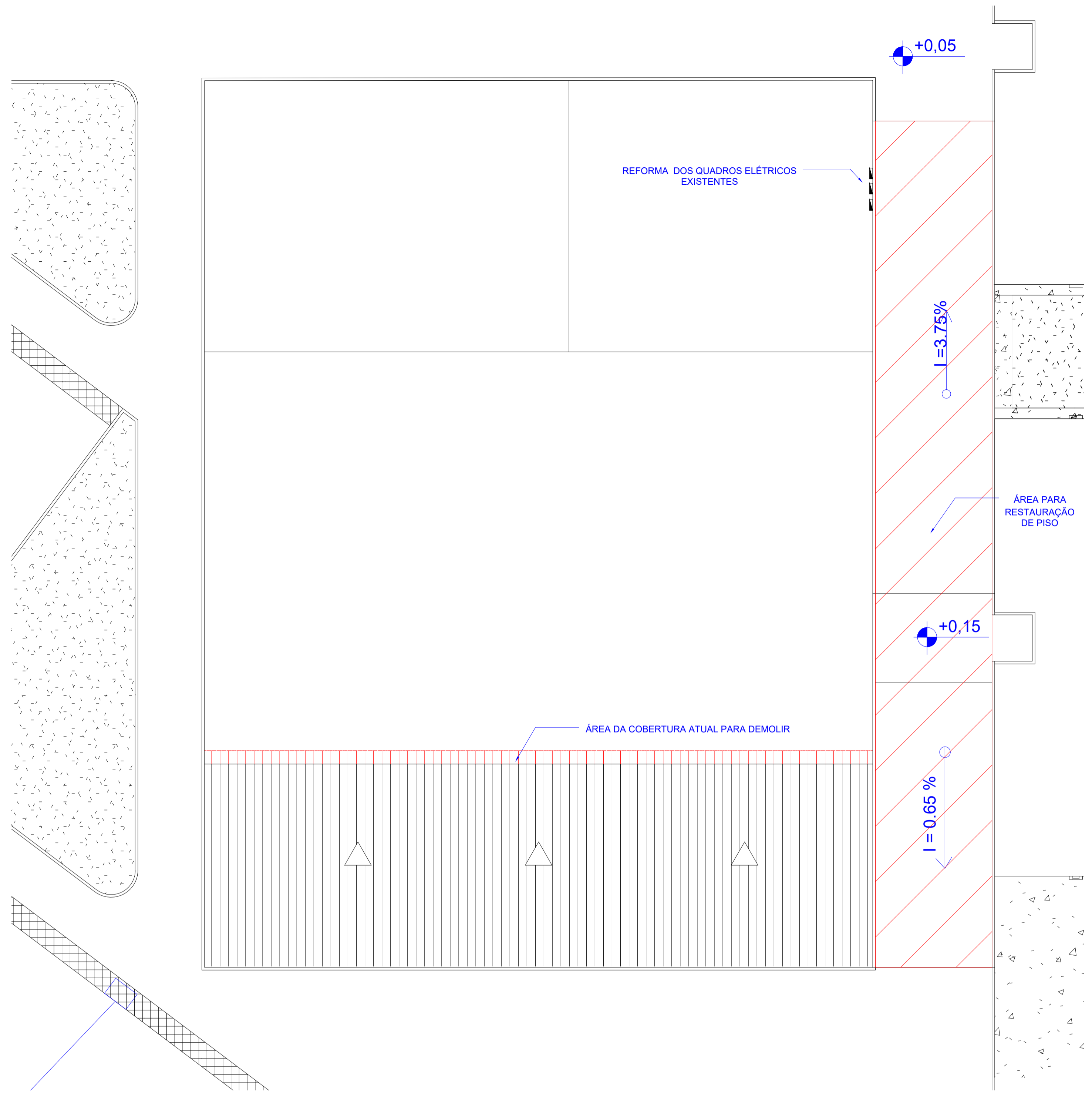
1 PLANTA BAIXA ATUAL
