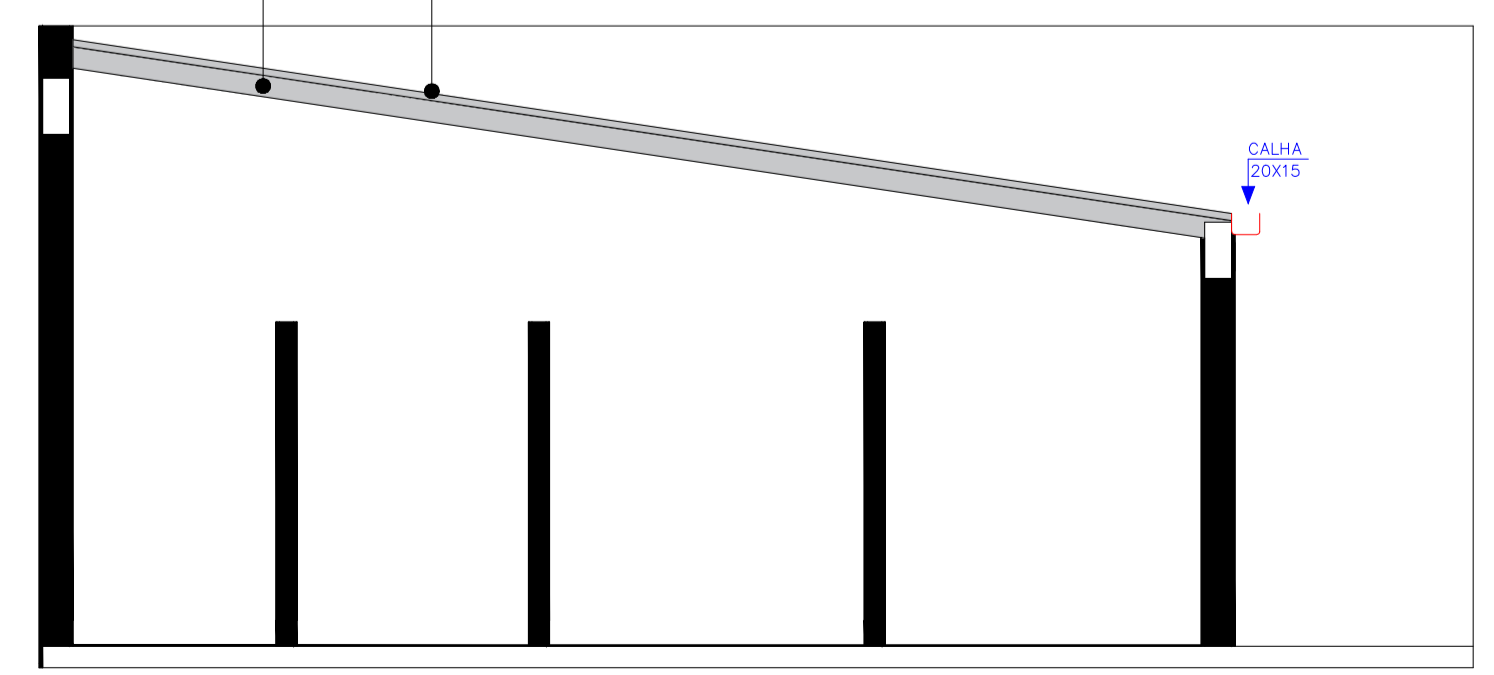
2 CORTE A ESCALA 1:25
